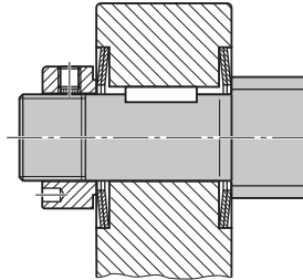
Serraggio con molla a disco
