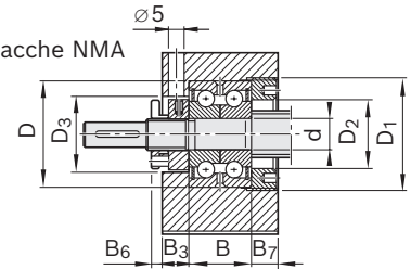
LGN-B-... con ghiera a tacche NMA
