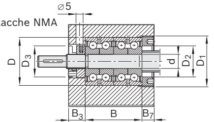
LGN-C-... con ghiera a tacche NMA
