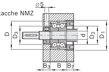
LGN-B-... con ghiera a tacche NMZ
