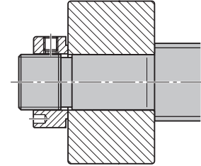
Serraggio fisso
