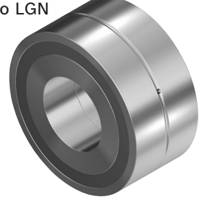
Cuscinetti di vincolo assiale a doppia corona di sfere a contatto obliquo LGN
