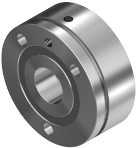
Rodamiento axial de contacto angular LGF
