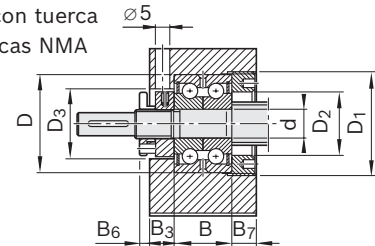
LGN-C...con tuerca con muescas NMA
