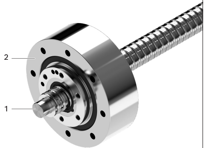
1 Husillo de husillo de bolas (BASA) 2 Tuerca accionada FAR
