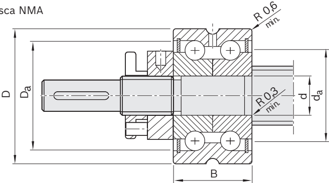
LGN-C-... con tuerca con muescas NMA
