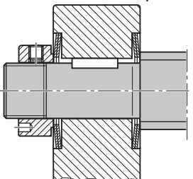
Sujeción con muelle de plato
