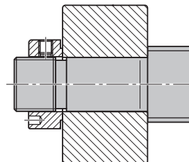
Sujeción fija
