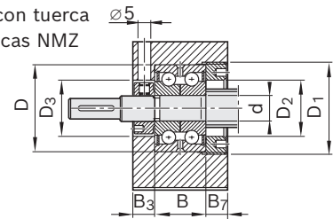
LGN-B...con tuerca con muescas NMA
