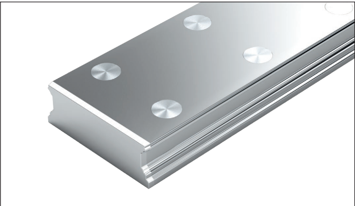
Raíles guía de bolas con tapones de acero
