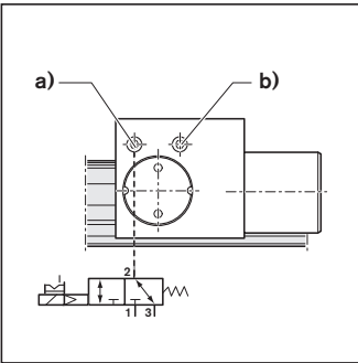
a) Conexión de aire b) Filtro de aire Diámetro nominal: Tamaños 15 - 20: mín. 4 mm Tamaños 25 - 65: mín. 6 mm
