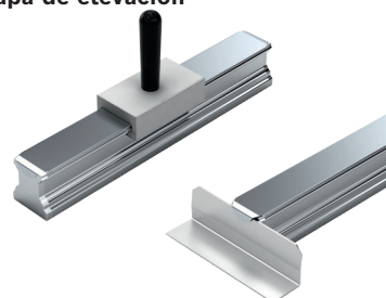
Juego de montaje para banda de protección con ayuda para el montaje y chapa de elevación
