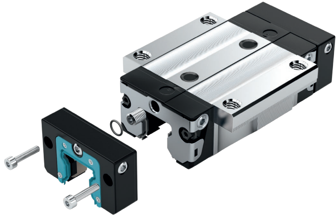
Patín de bolas estándar con dos unidades de lubricación adicional
