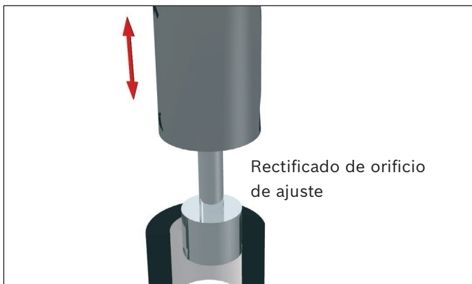
Rectificado redondo interior
