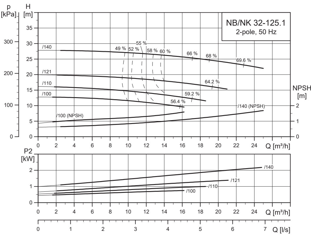
NB, NK 32-125
