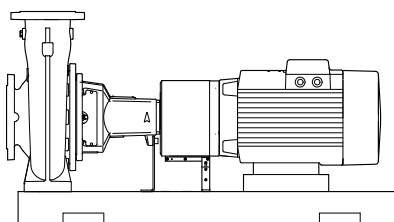
Fig. 19 Vista schematica dell'unità pompa/motore NK montata su un basamento
