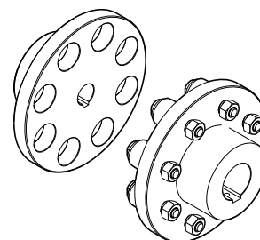
Fig. 16 Giunto standard
