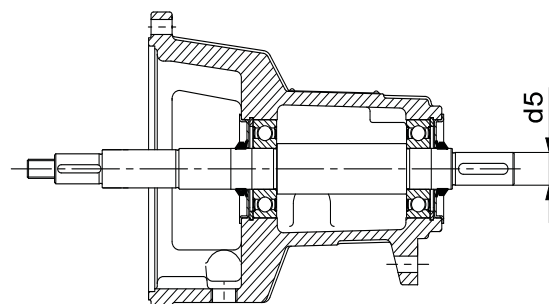
Fig. 10 Staffa di supporto ed albero
